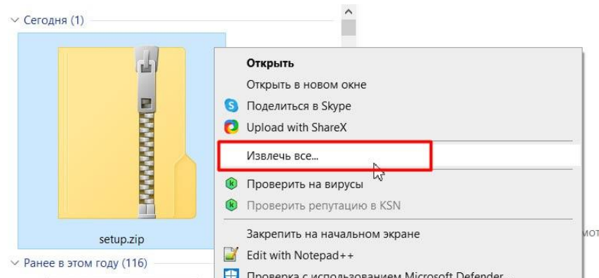
Рисунок 2.3. — Разархивирование файлов.
